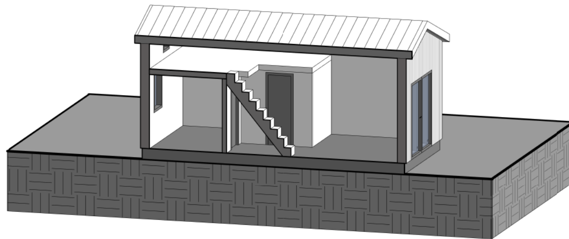
3D- SEKTION
