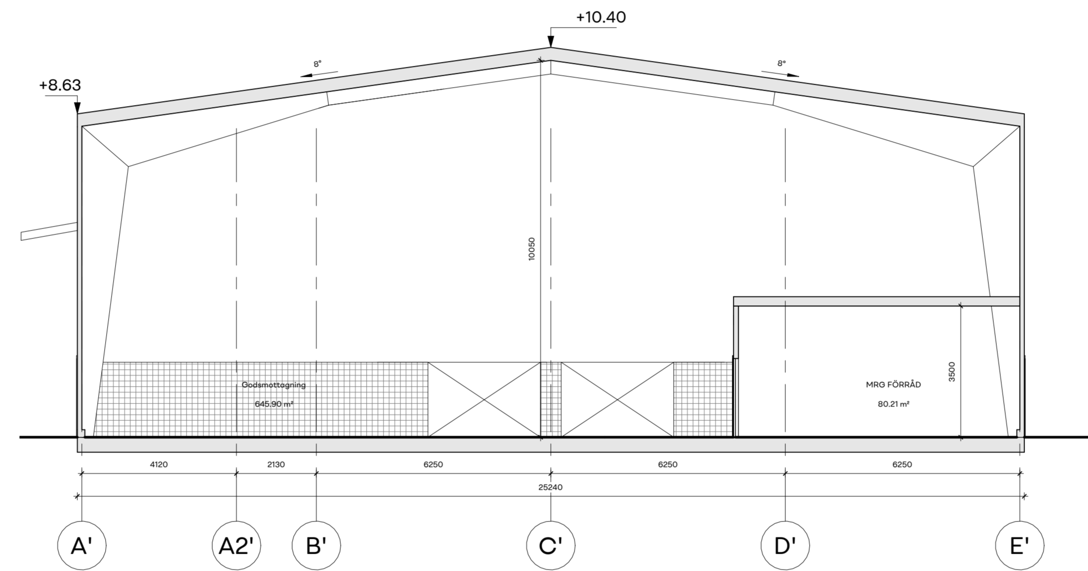
A SEKTION A-A 1:100
