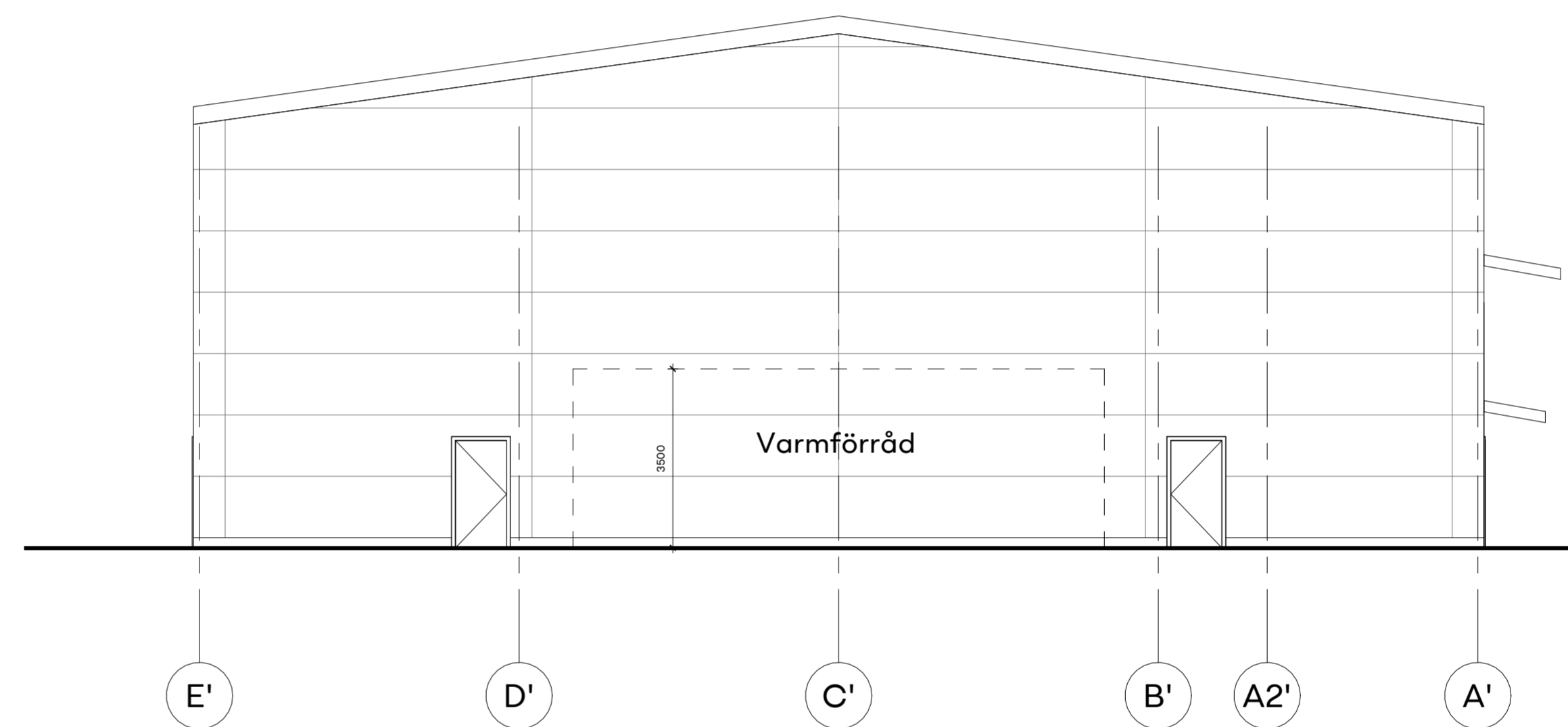
3 ÖST 1:100
