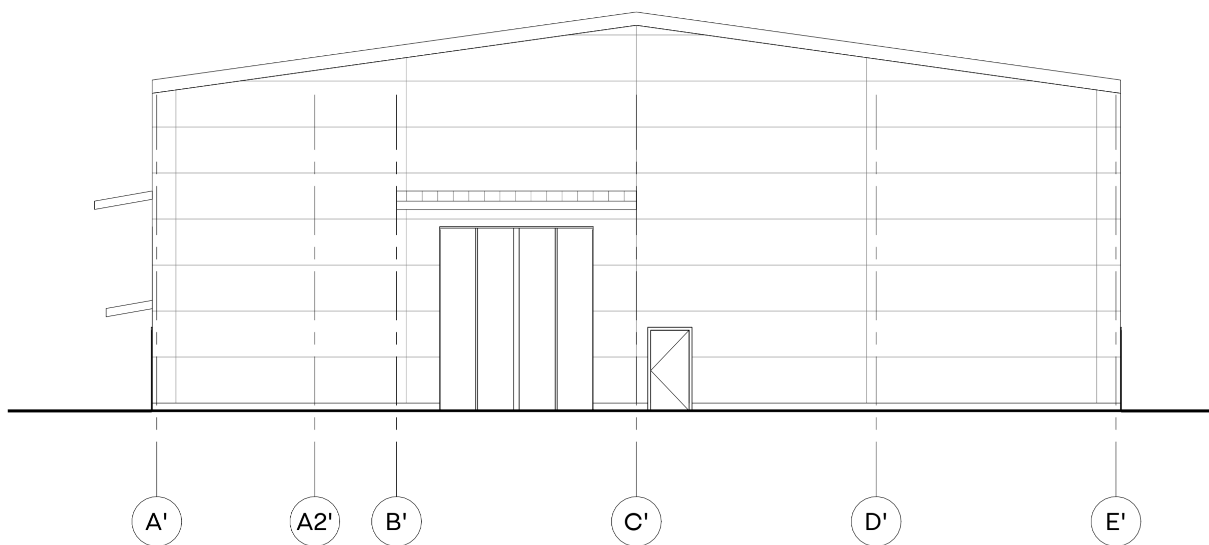
2 VÄST 1:100
