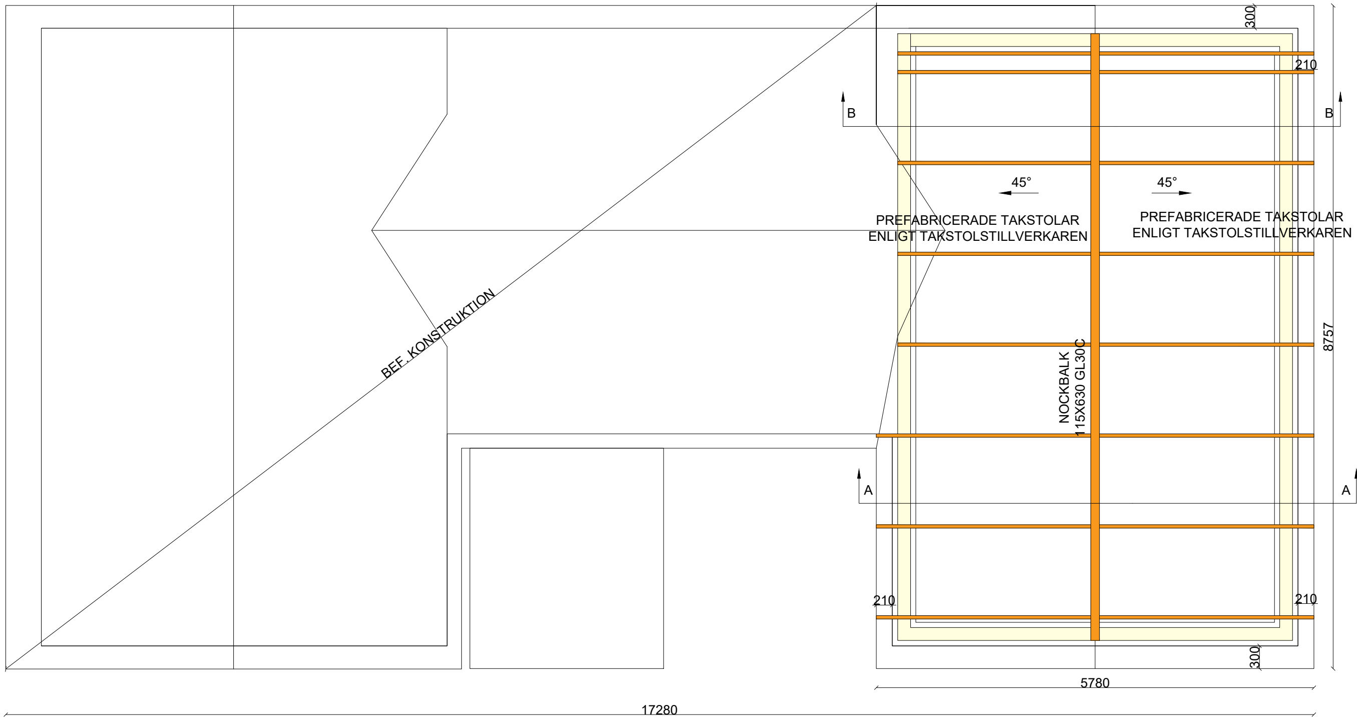
TAKPLAN 1:50
