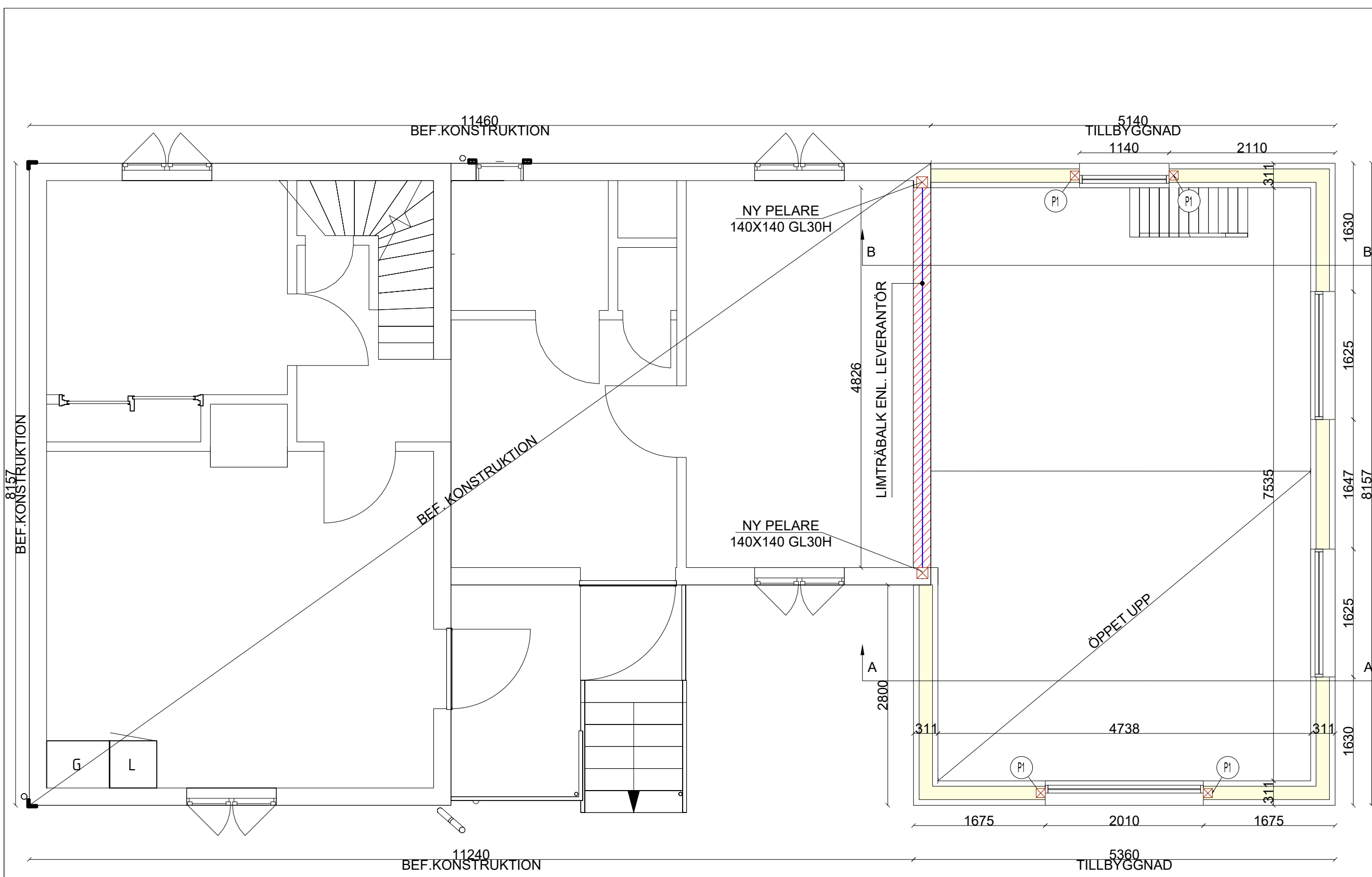
ENTRÉPLAN 1:50
