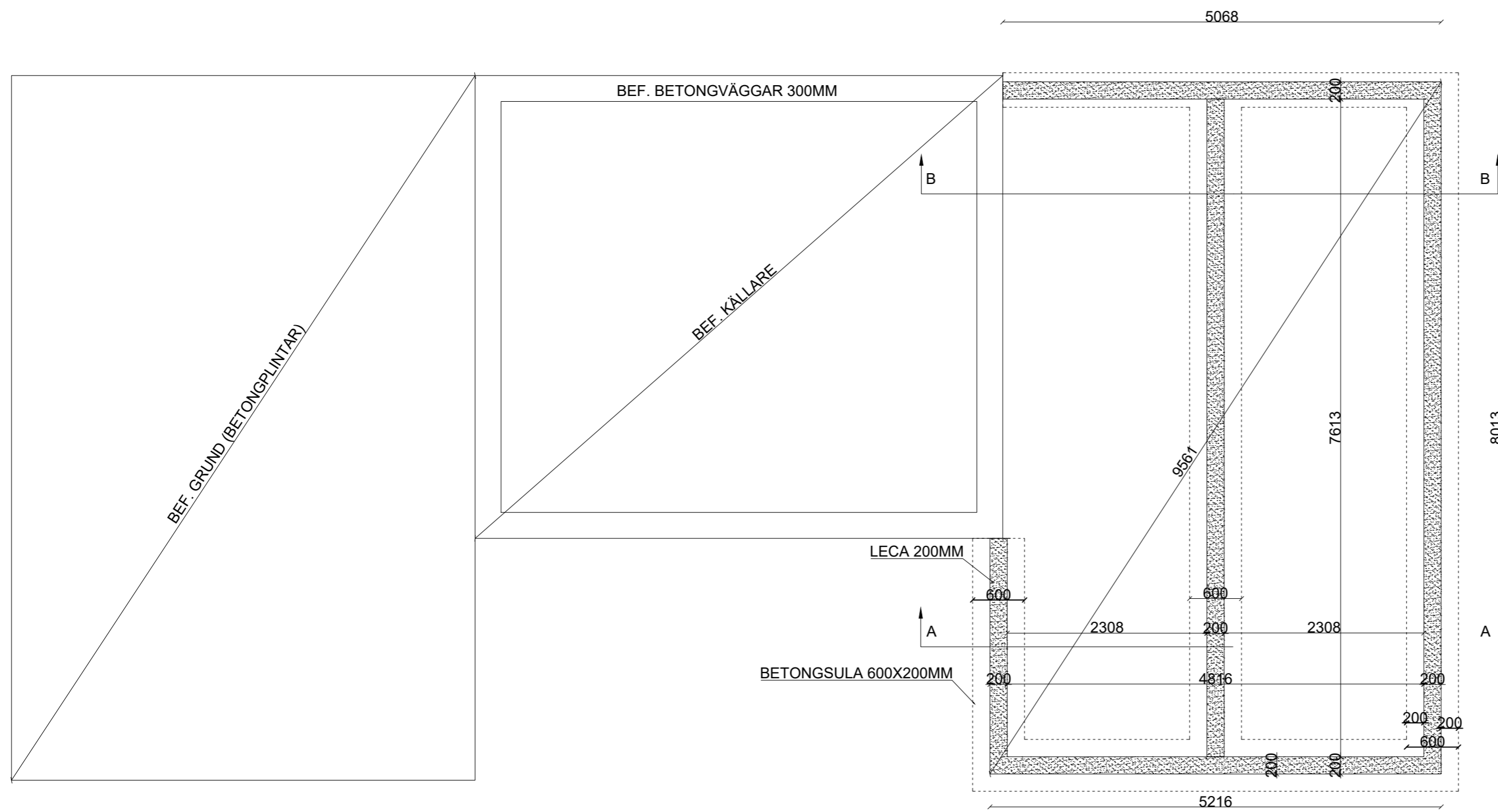
GRUNDPLAN 1:50
