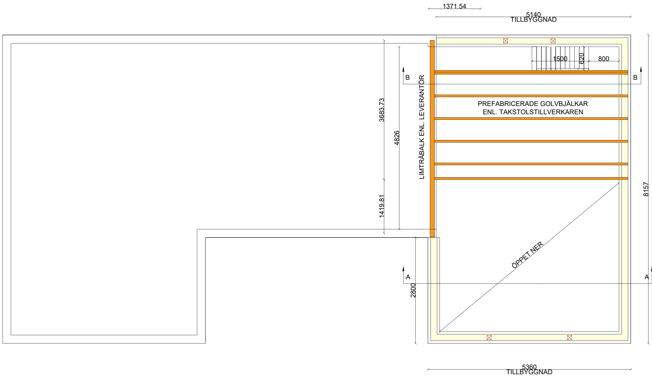
MELLANBJÄKLAG 1:50
