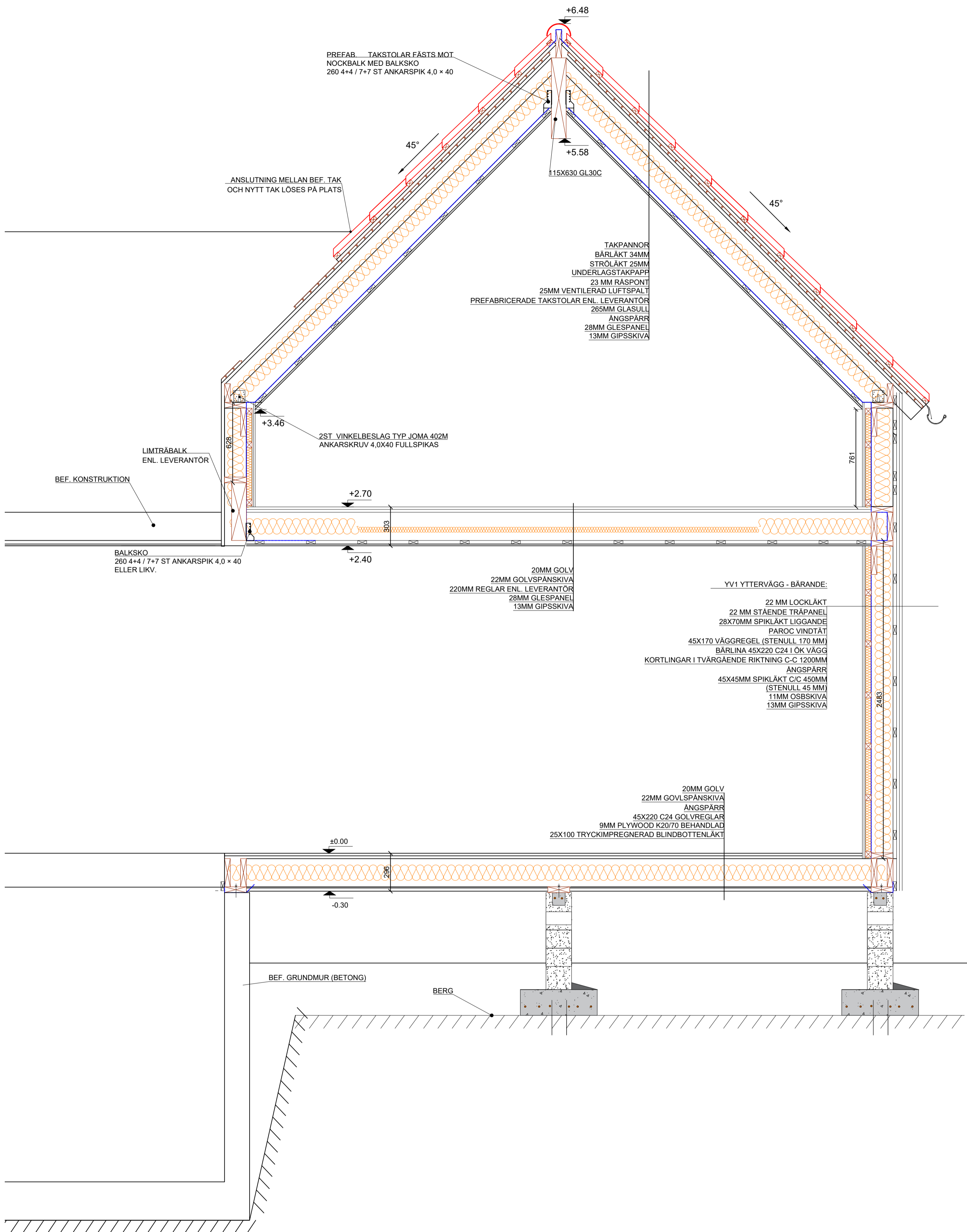
Sektion B-B 1:20
